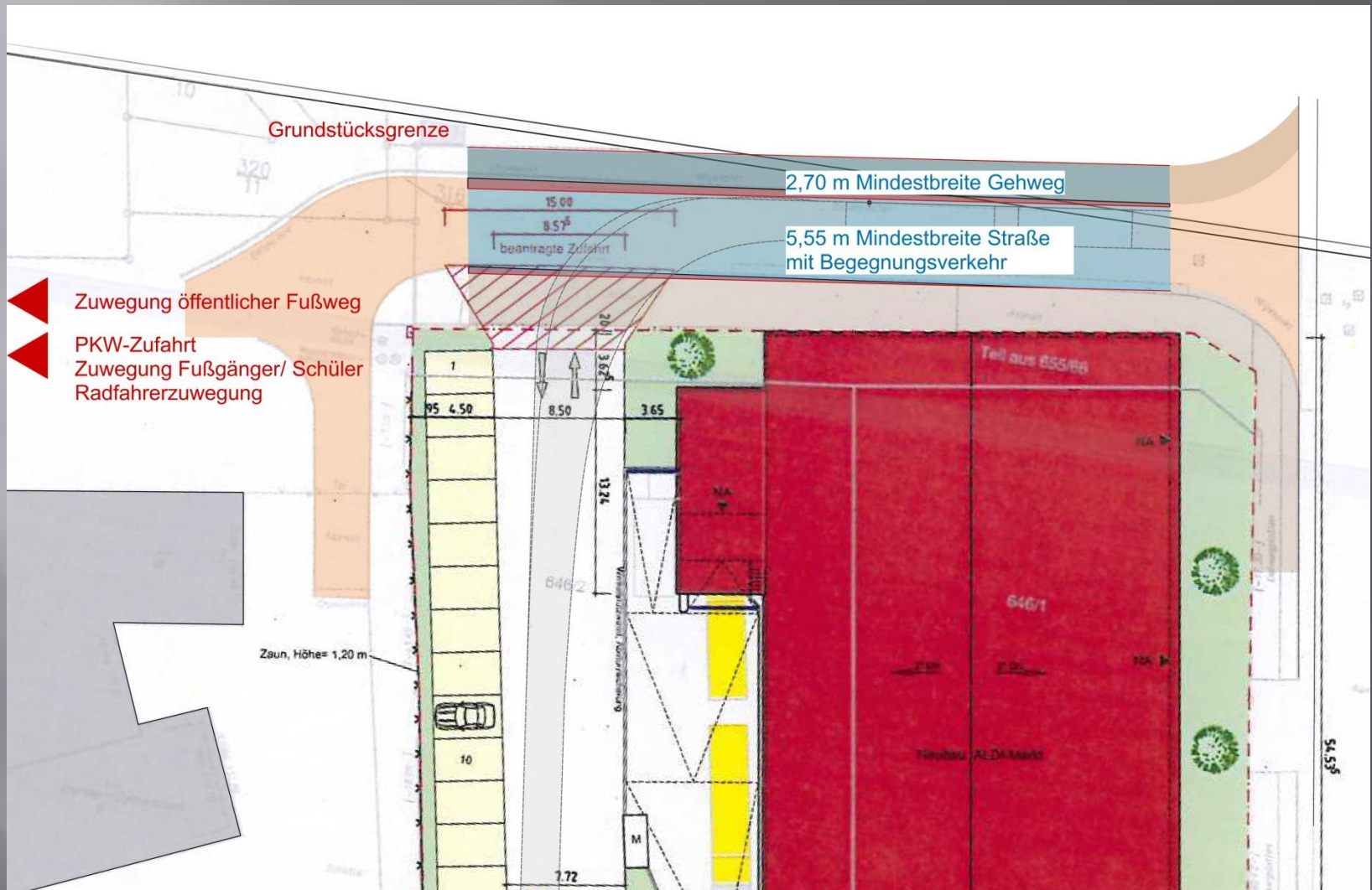
Mindestbreiten / Differenzen / Engpass
