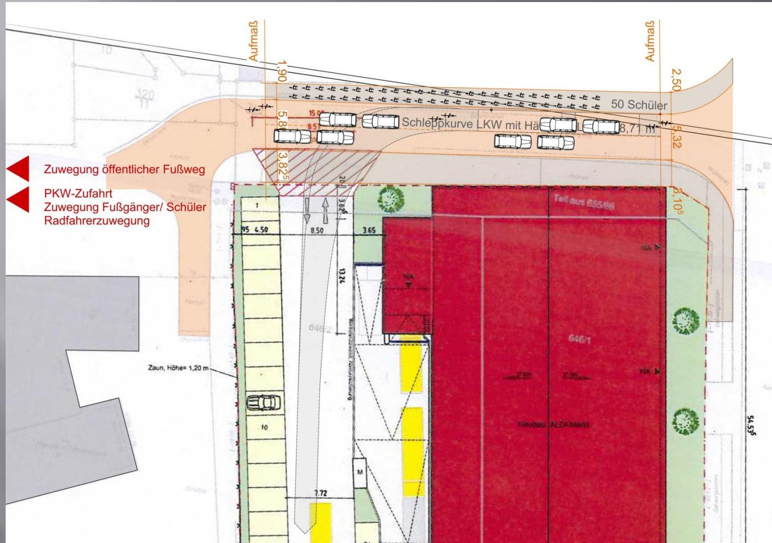
Nutzung durch 50 Schüler sowie PKW und Radfahrer
