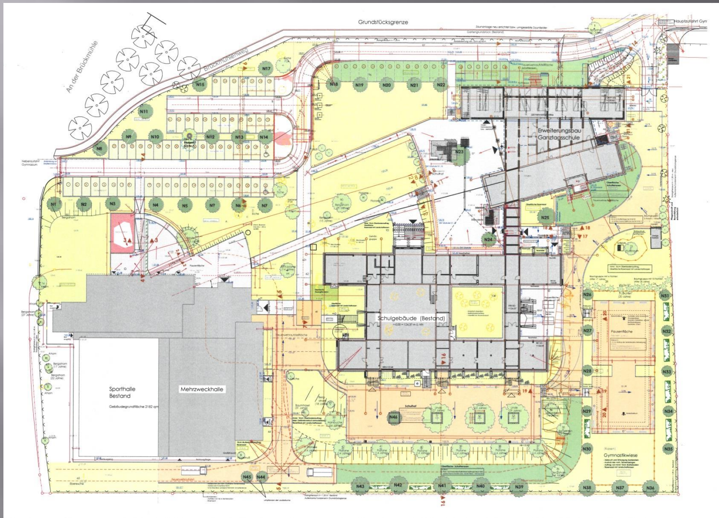
Lageplan Schulgelände J.-G.-Herder Gymnasium
