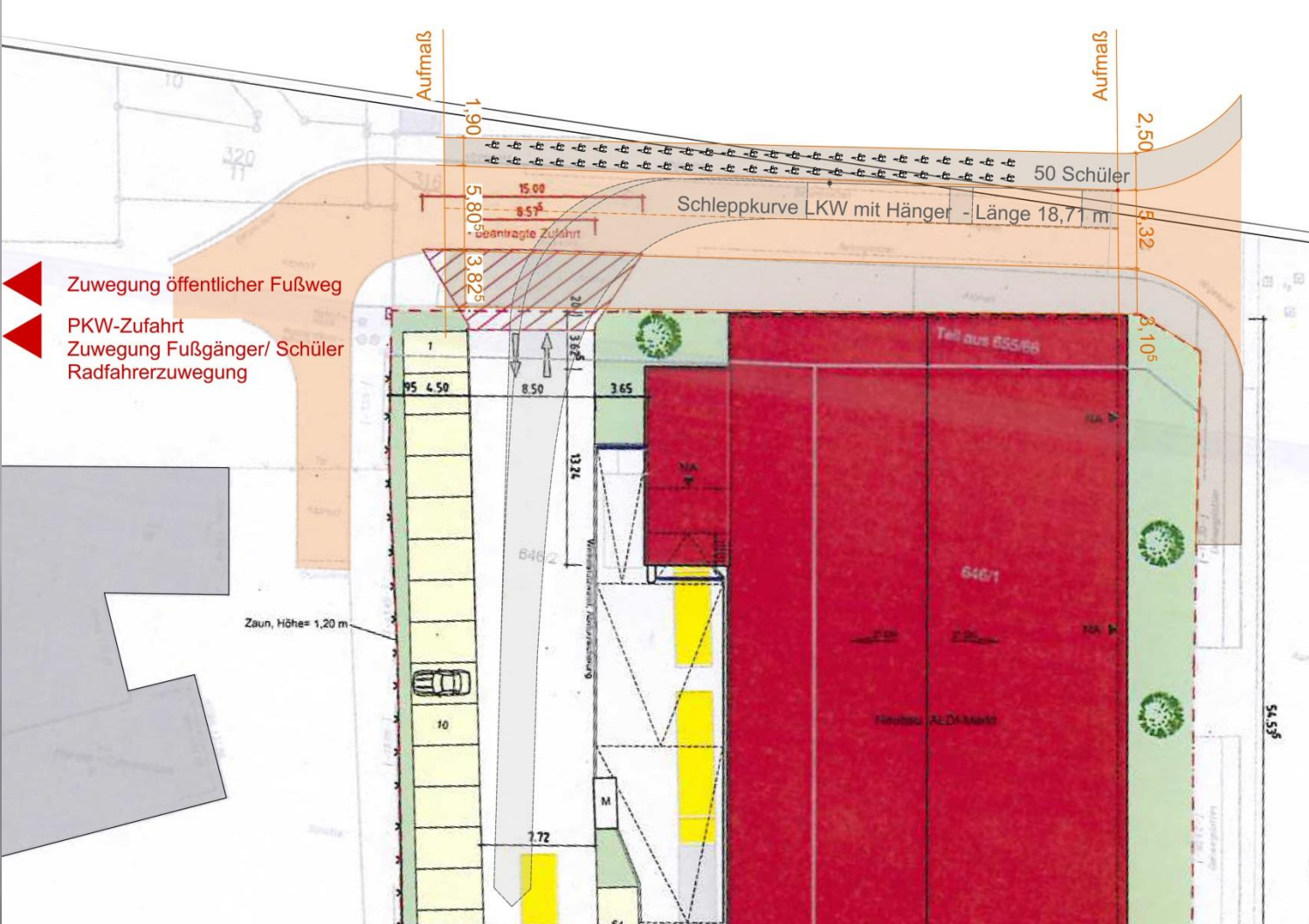
Fußwegnutzung durch 50 Schüler
