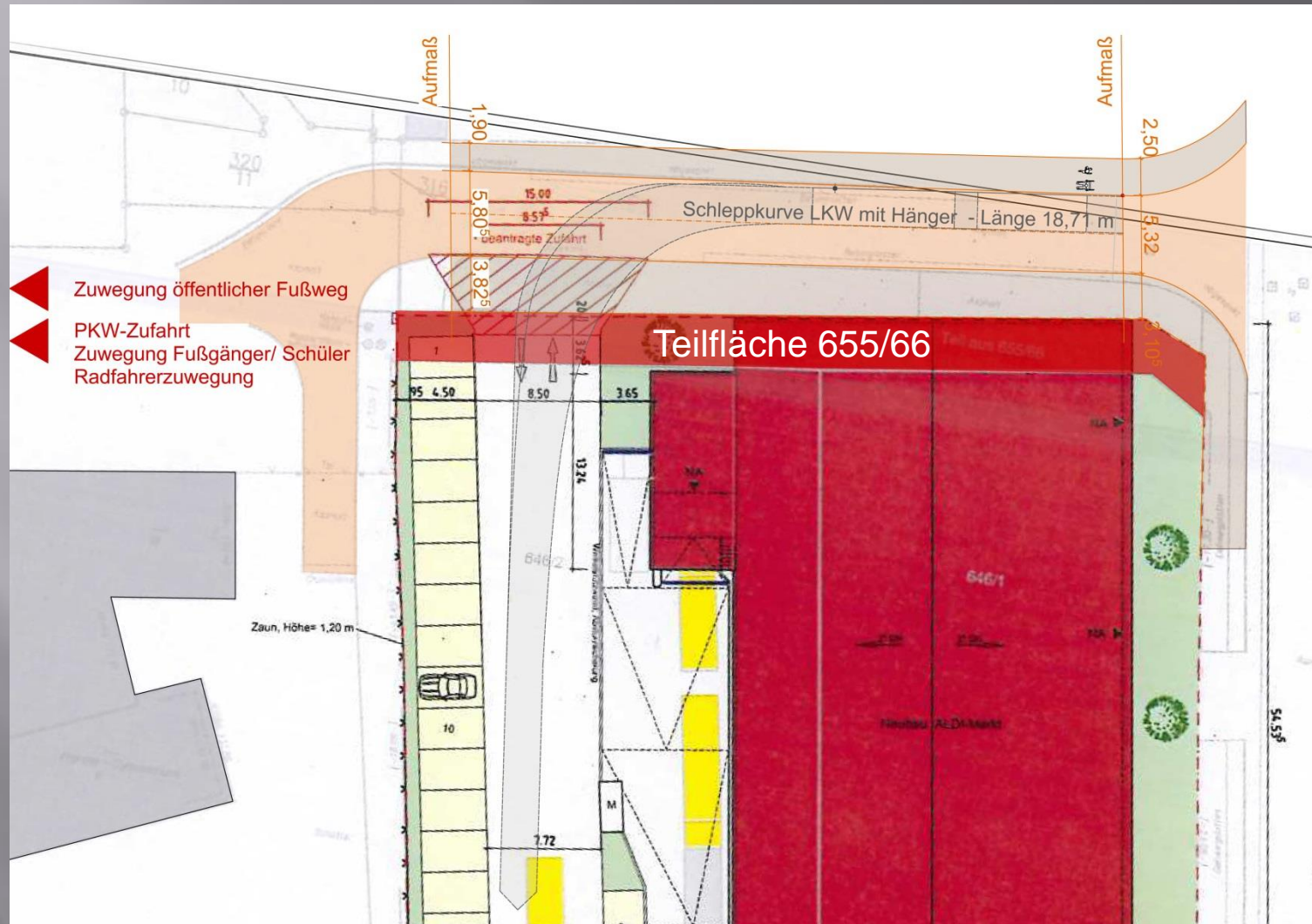
Lageplan mit Eintragung Grenzverschiebung Verschärfung der Engstelle durch Grundstücksübertrag
